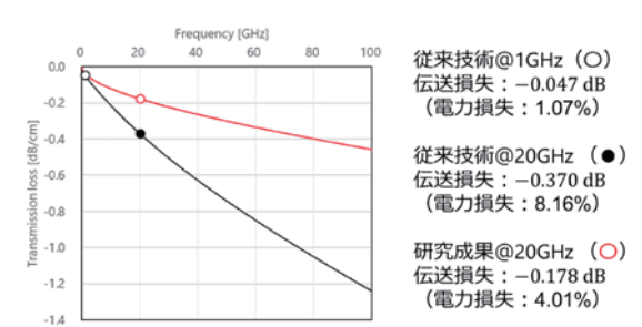
開発材料及び分子接合剤での平滑面接着時の伝送損失計算結果
