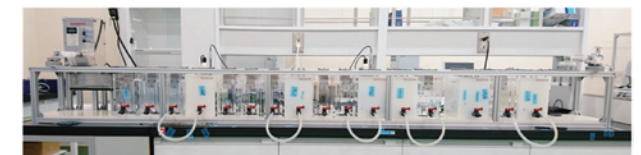
ロール to ロールめっき装置全景
